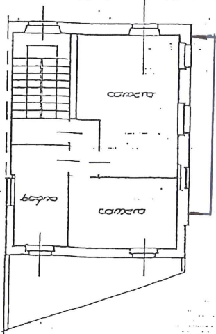
PIANO PRIMO 11-210
